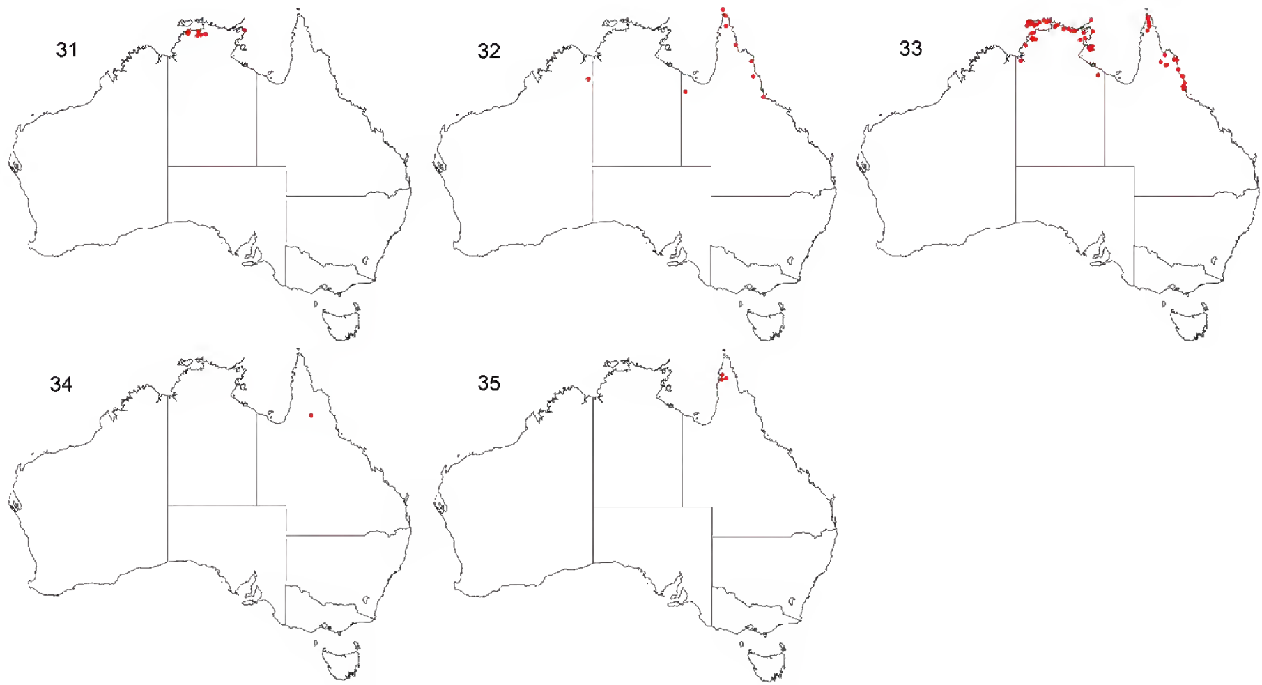
Fig. 13. Distribution maps: 31. E. tricornum ; 32. E. truncatum ; 33. E. willdenovianum ; 34. E. wolseleyi ; 35. E. zollingerianum .
